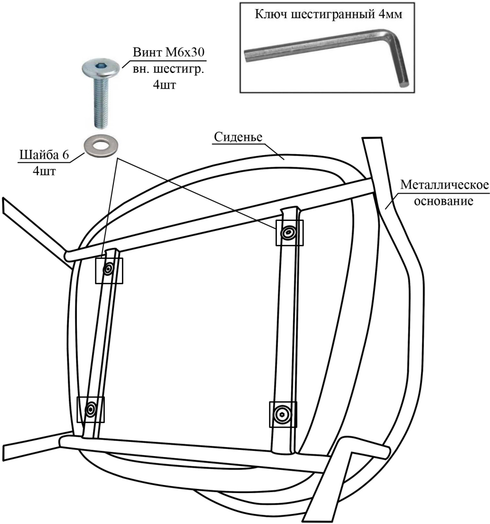
Сборка стула. Вид снизу
